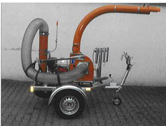
Laubverladegebläse Typ F 625 / Spezialausführung
