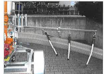
Klappbarer Ausleger für Schlauchführung
